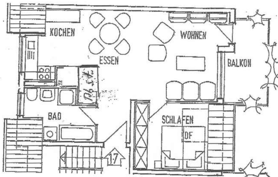
Grundriss
